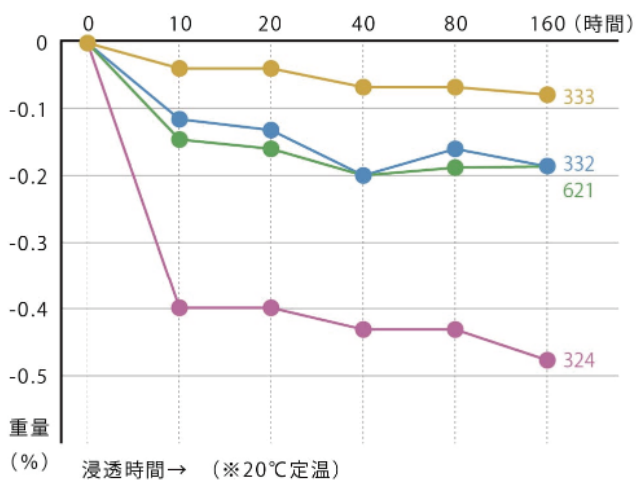
硝酸：20%重量変化
