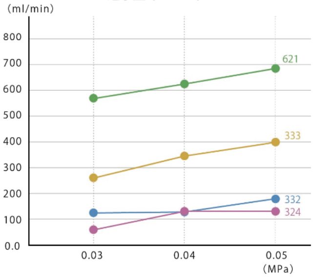
通水量 (水温20°C)
