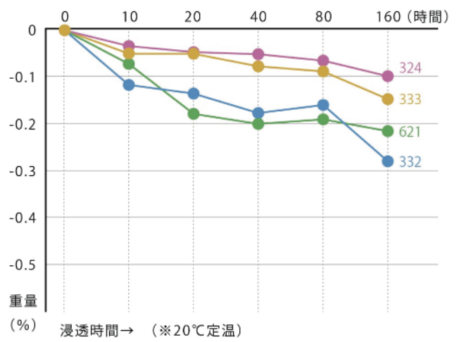
水酸化ナトリウム：20%重量変化
